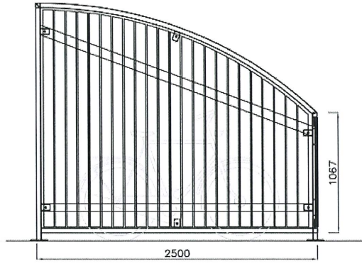
Rechterzijgezicht
