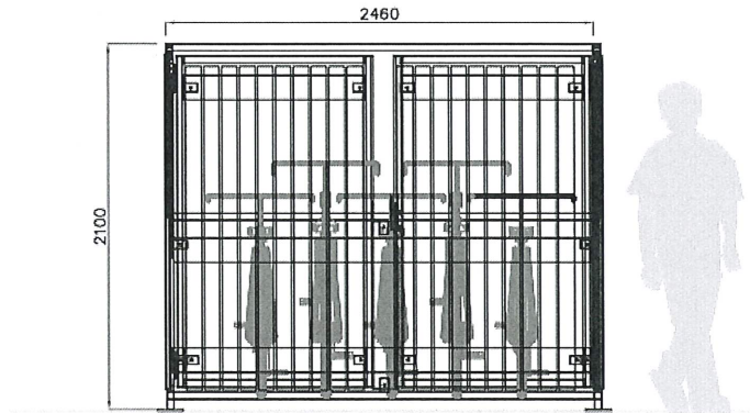
Vooraanzicht
