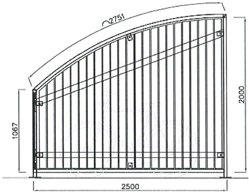
Linkerzijgezicht
